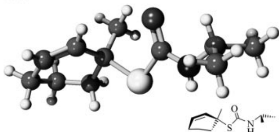
( - )-( S )- 20b
